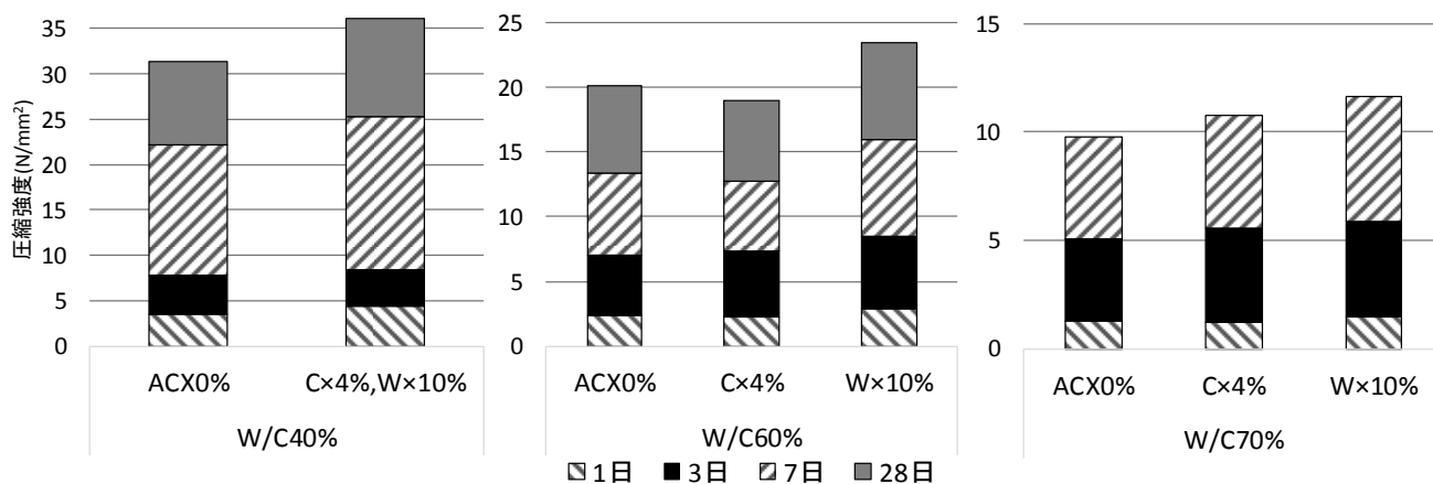
図-2 圧縮強度試験結果
