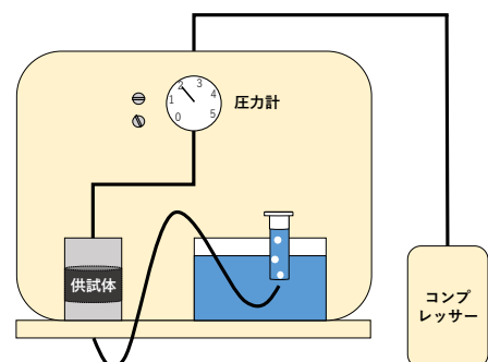
図-1 透気試験の概略
