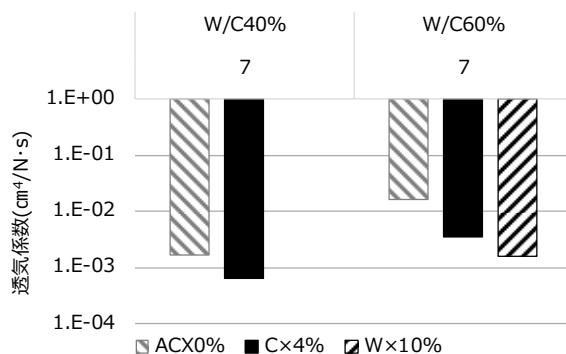
図-3 透気係数測定結果
